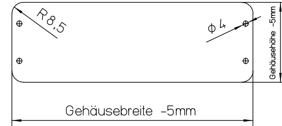
Frontplatte-Rückplatte
