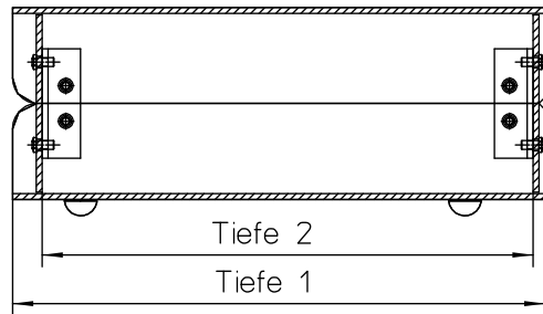
Gehäuse Prinzipskizze
