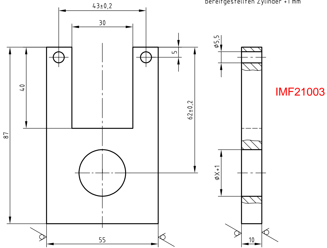
Skizze 2 \sqrt{Rz\ 16} ( \checkmark )
