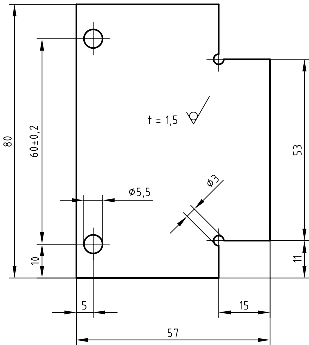
Skizze 7 \sqrt{Rz\ 16} ( \checkmark )
