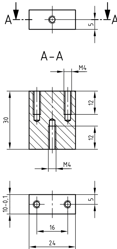
Skizze 8 \sqrt{Rz\ 16}
