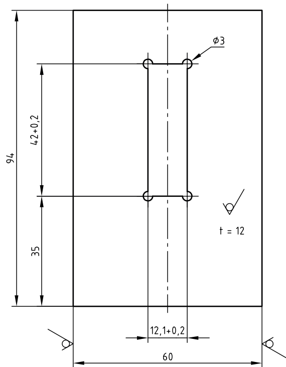
Skizze 1 \sqrt{Rz\ 16} (✓)
