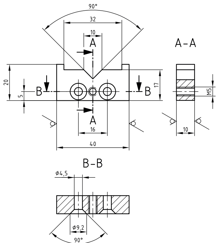
Skizze 4 \sqrt{Rz\ 16} (✓)
