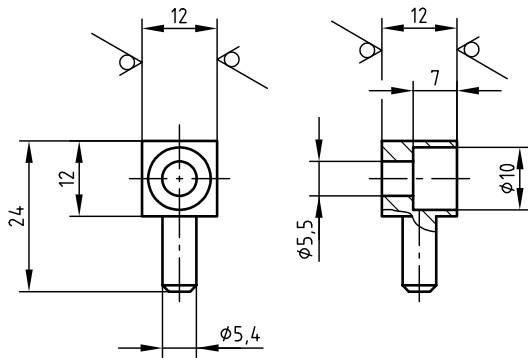
Skizze 7 \sqrt{Rz\ 16} (✓)
