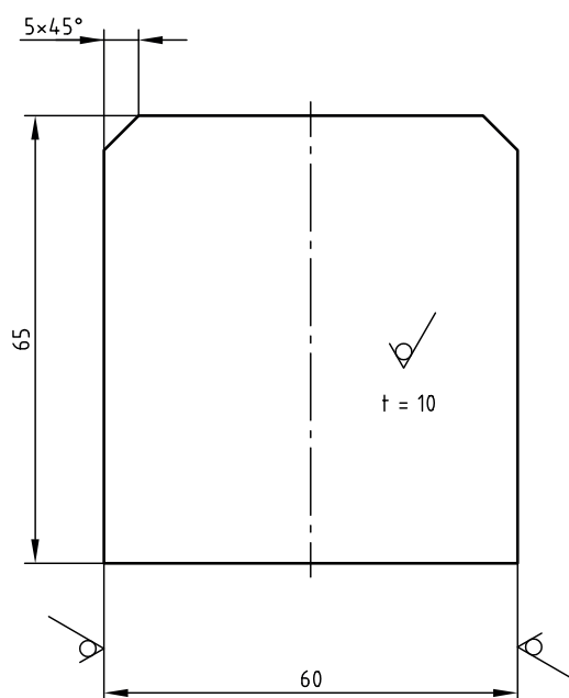
Skizze 3 \sqrt{Rz\ 16} (✓)
