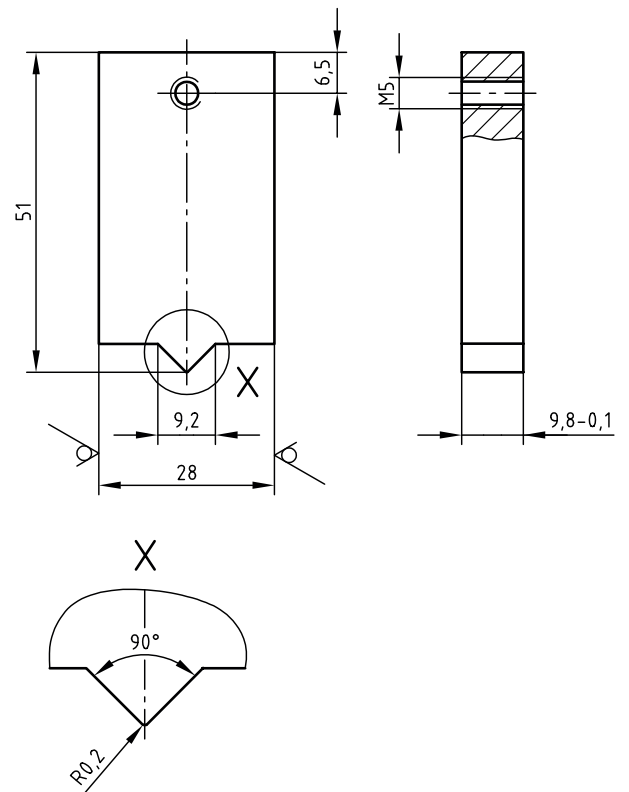
Skizze 4 \sqrt{Rz\ 16} (✓)
