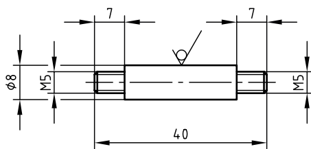
Skizze 9 \sqrt{Rz\ 16} (✓)
