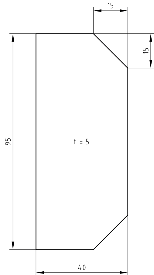
Skizze 2 Fl 40×5-95
