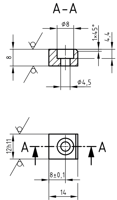
Skizze 4 \sqrt{Rz\ 16} ( \checkmark )
