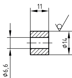
Skizze 5 \sqrt{Rz\ 16} ( \checkmark )
