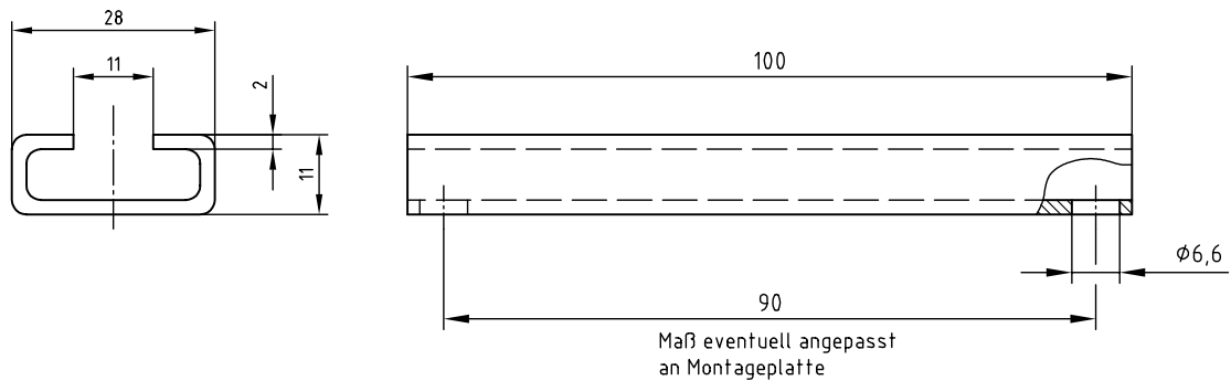
Skizze: Tragschiene
