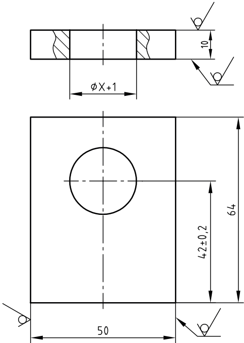
Skizze 4 \sqrt{Rz\ 16} ( \checkmark )
