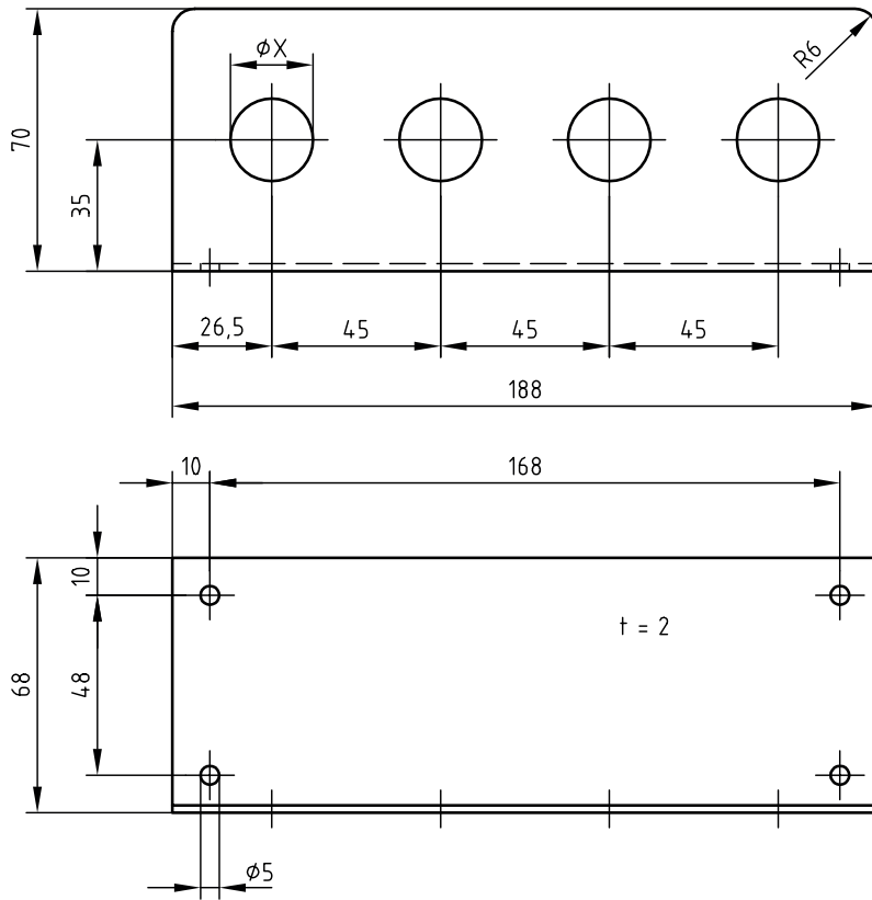
Skizze: Montagewinkel für elektrische Signalgeber
