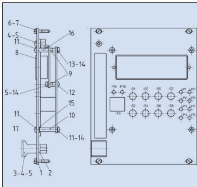
Bausatz Einschub 5035-1363
