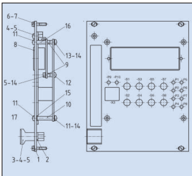
Bausatz Einschub 5035-1363
