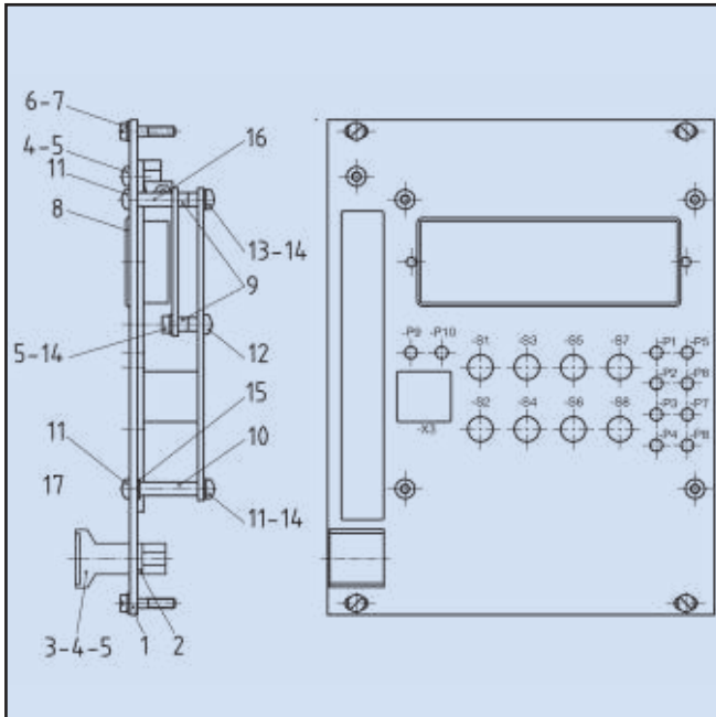
Bausatz Einschub 5035-1363
