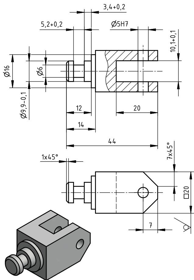
Skizze C \sqrt{Rz\ 16} ( \checkmark )
