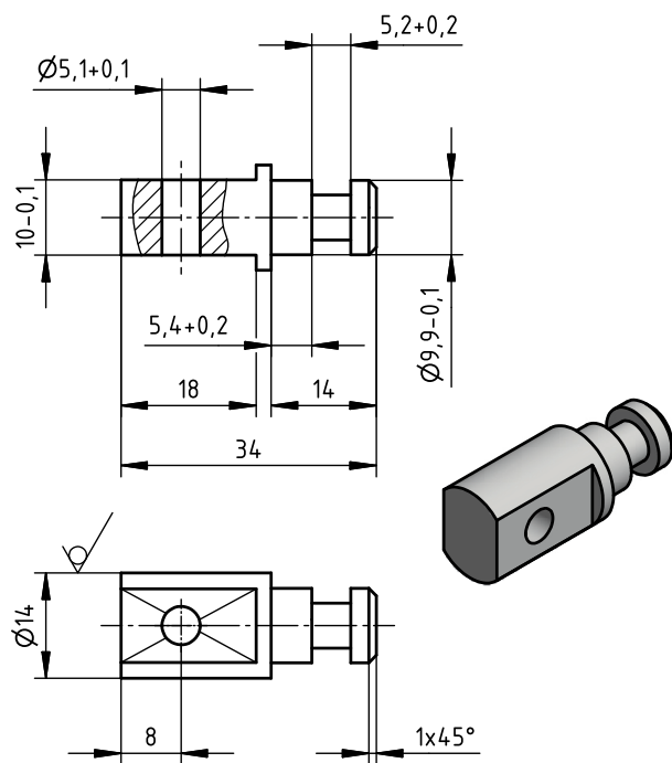
Skizze D \sqrt{Rz\ 16} ( \checkmark )
