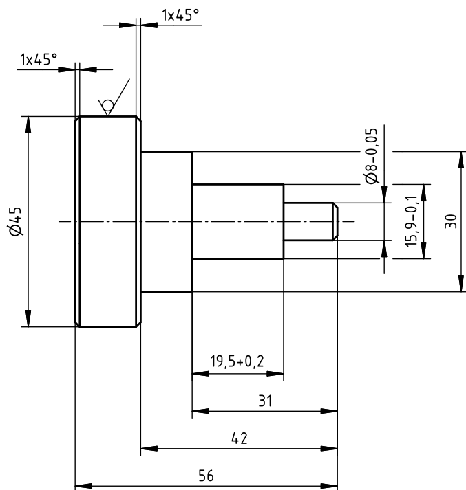
Skizze E \sqrt{Rz\ 16} ( \checkmark )
