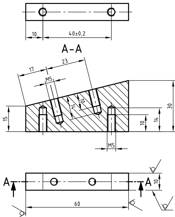
Skizze 1 \sqrt{Rz\ 16} ( \checkmark )
