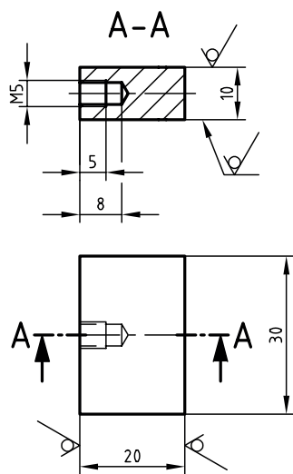
Skizze 3 \sqrt{Rz\ 16} ( \checkmark )
