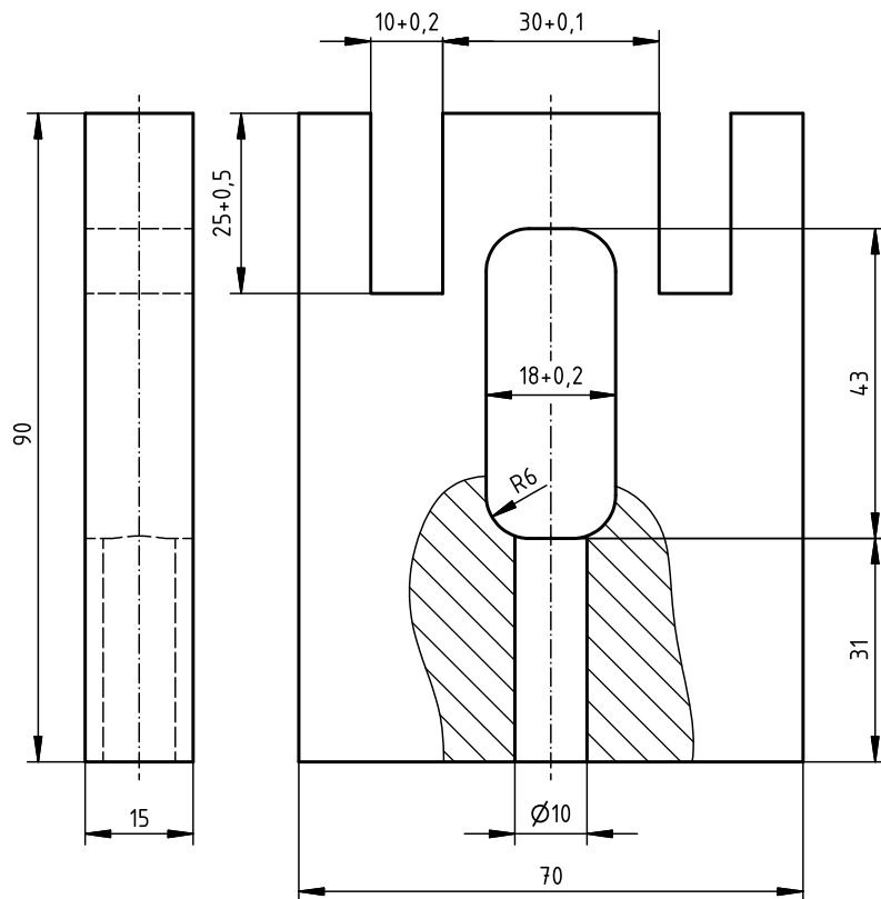
Skizze 1 \sqrt{Rz\ 16} (✓)
