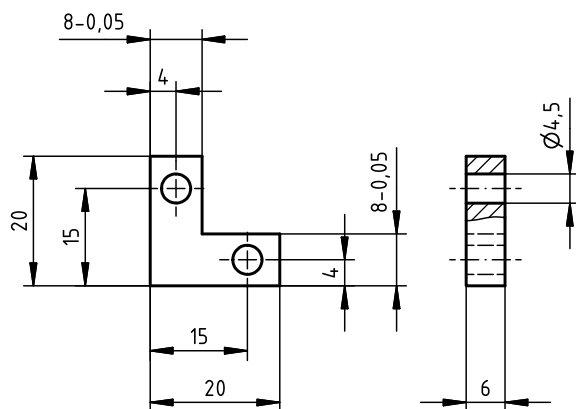
Skizze 3 \sqrt{Rz\ 16} (✓) 2 Stück
