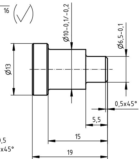
Skizze 9 \sqrt{Rz\ 16} (✓)
