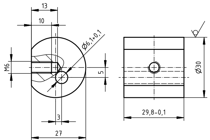
Skizze 6 \sqrt{Rz\ 16} (✓)
