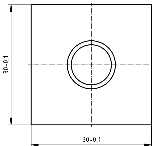
Skizze 8 \sqrt{Rz\ 16} (✓)
