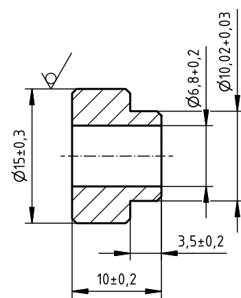
Skizze 9 \sqrt{Rz\ 16} (✓)
