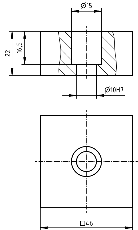
Skizze 2 \sqrt{Rz\ 16} (✓)
