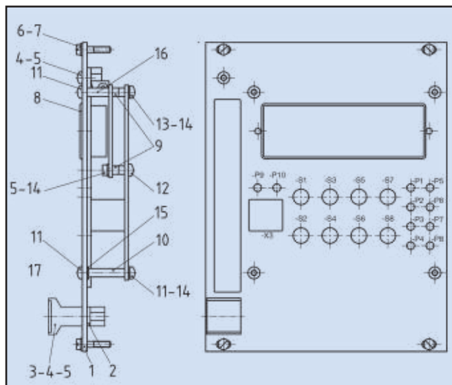
Bausatz Einschub 5035-1363
