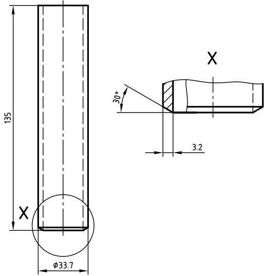
Skizze 1 2 Stück
