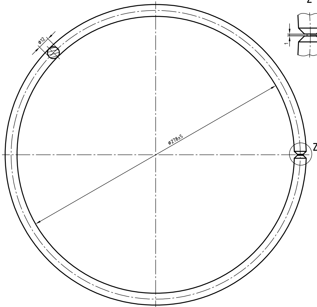
Skizze 4 Biegeklötz
