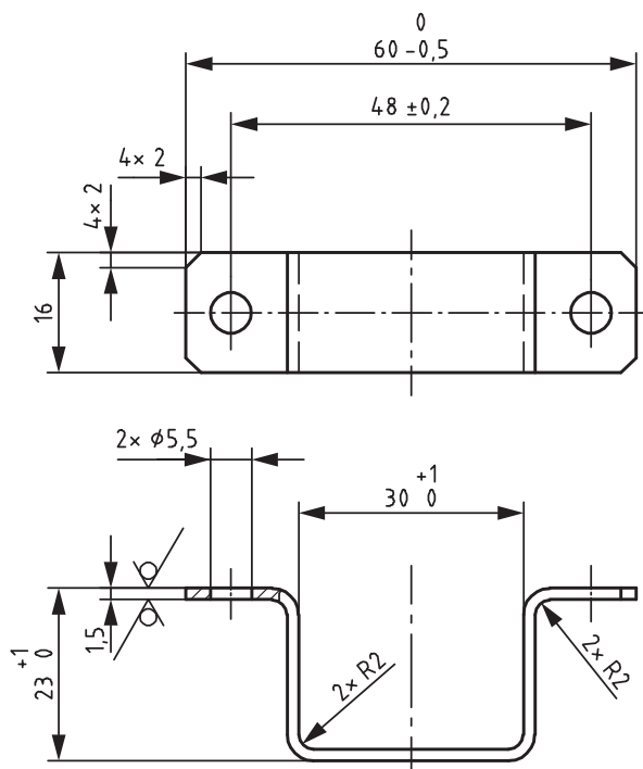
Skizze 3 \sqrt{Rz\ 16} (✓)
