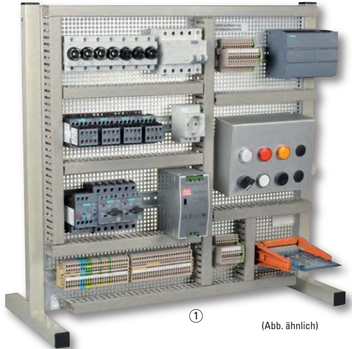
Frühjahr 2024 Platine Prozesssimulation 5035-1449
