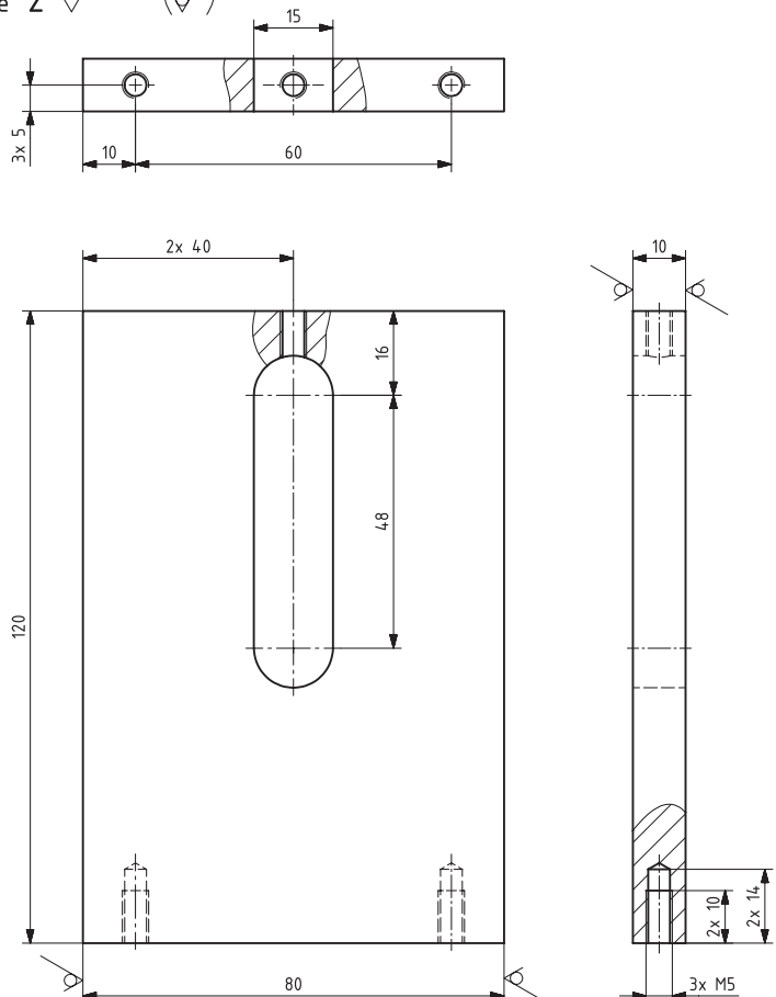
Skizze 2 \sqrt{Rz\ 16} ( \checkmark )
