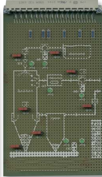
Frühjahr 2022 Platine Prozesssimulation 5035-1402
