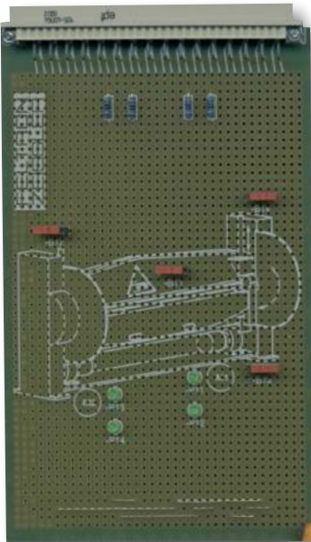
Frühjahr 2023 Platine Prozesssimulation 5035-1429
