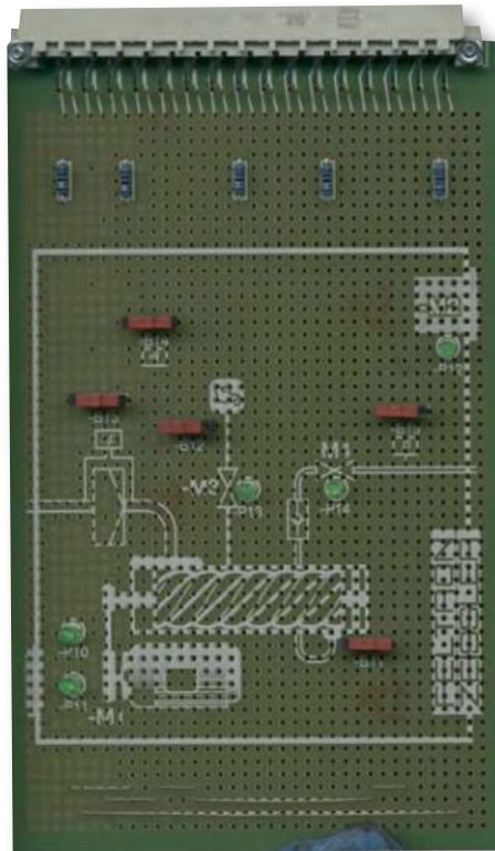
Frühjahr 2024 Platine Prozesssimulation 5035-1449
