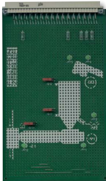
Herbst 2021 Platine Prozesssimulation 5035-1393
