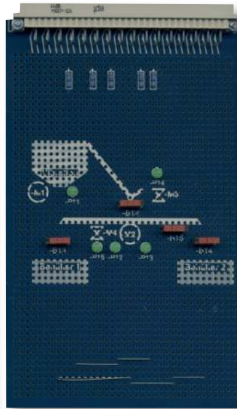
Frühjahr 2021 Platine Prozesssimulation 5035-1388
