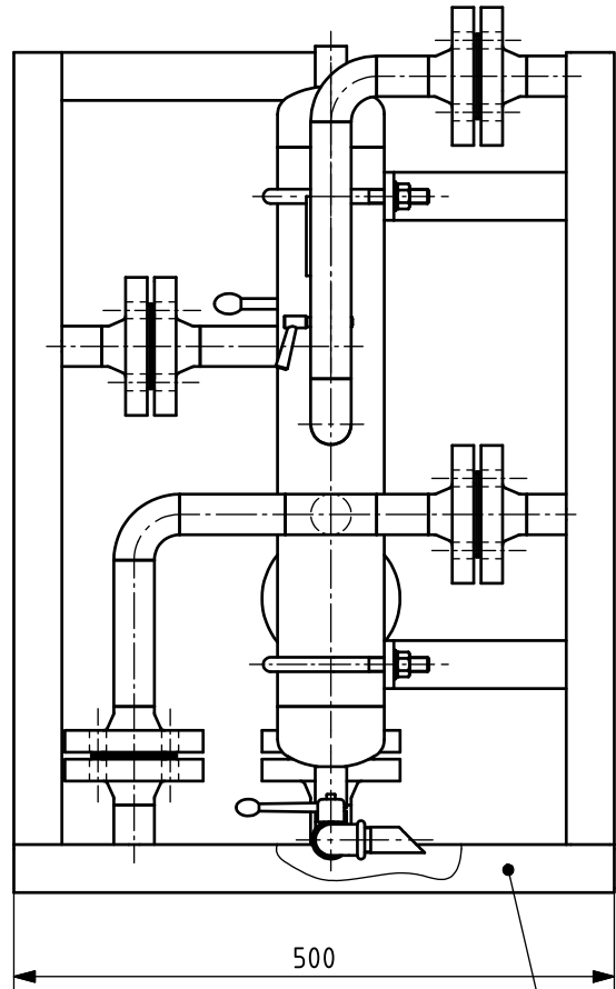
Standard-Einbaugestell
