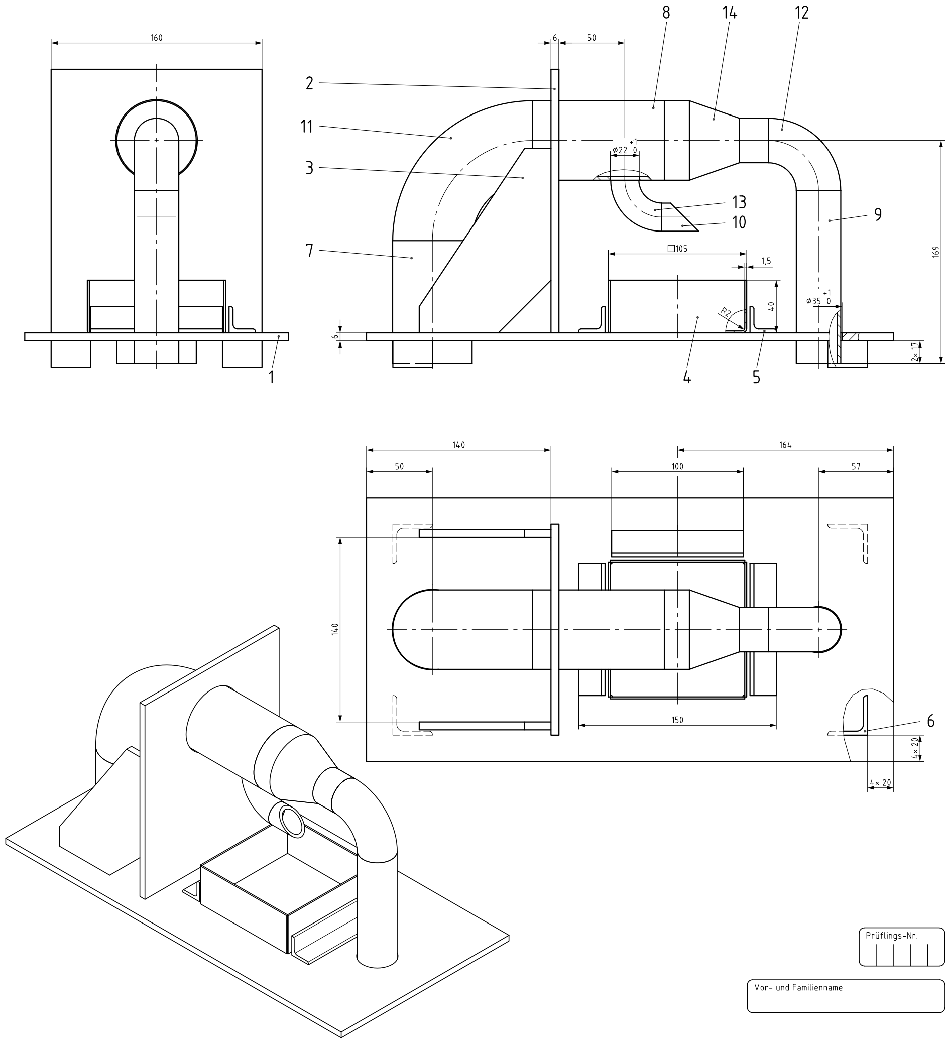
Allgemeintoleranz für Schweißkonstruktionen nach DIN EN ISO 13920
