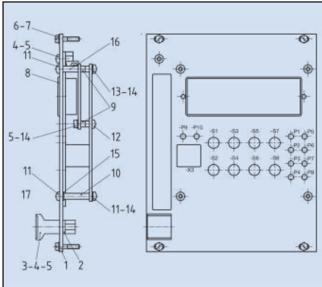
Bausatz Einschub 5035-1363
