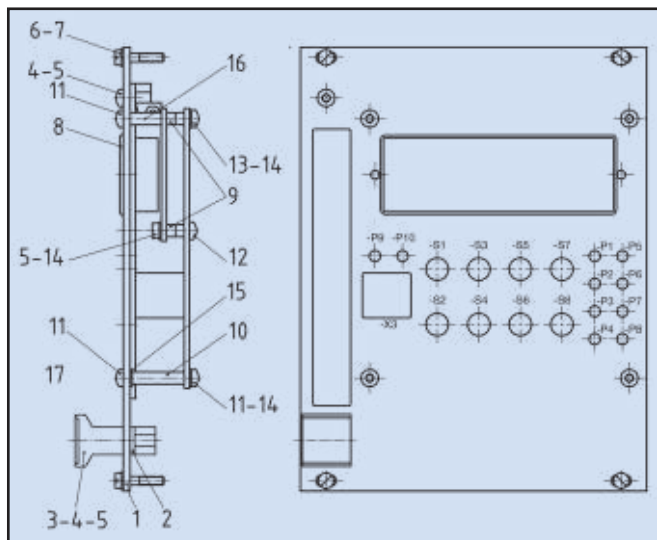
Bausatz Einschub 5035-1363
