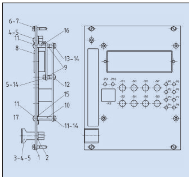
Bausatz Einschub 5035-1363
