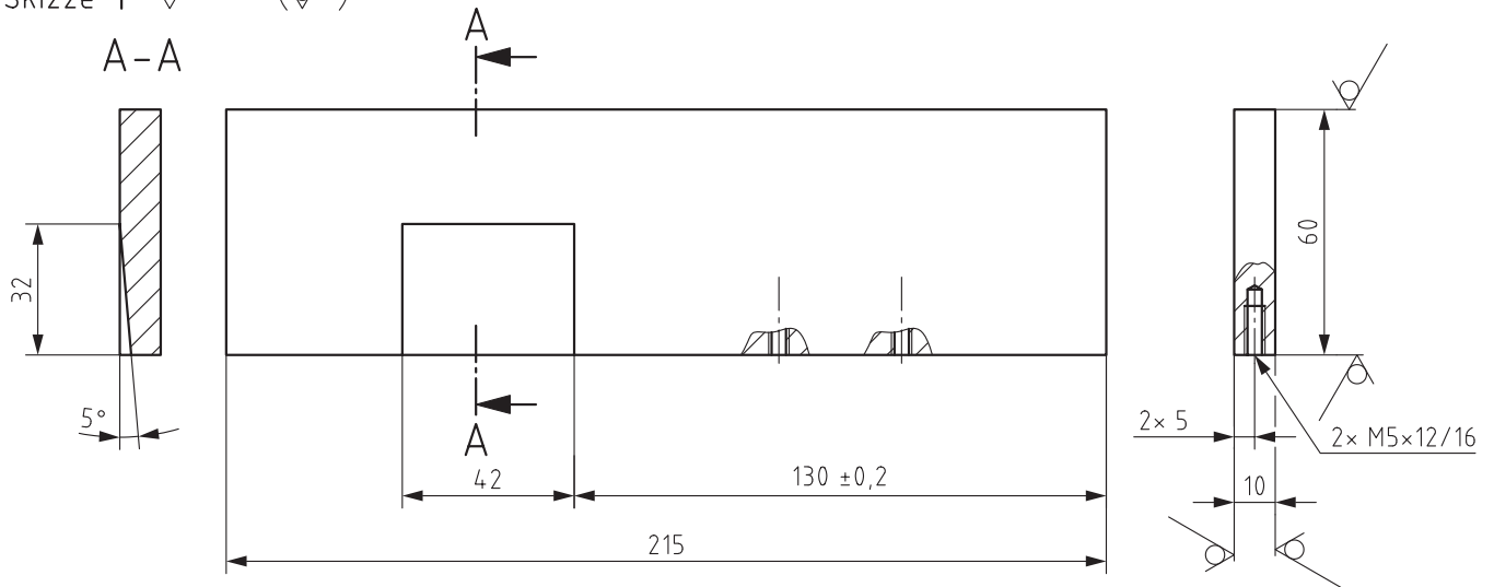
Skizze 2 \sqrt{Rz\ 16} (✓)
