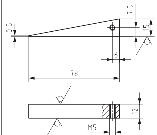
Skizze 5 \sqrt{Rz\ 16} (✓)
