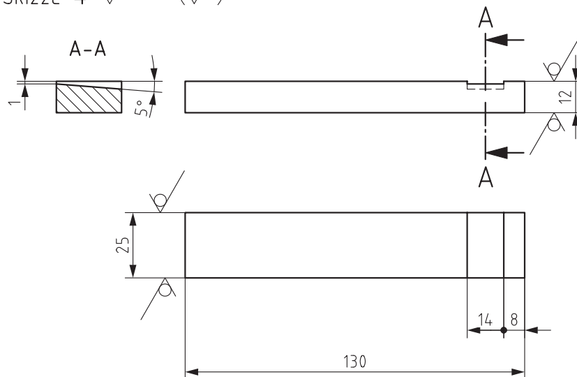
Skizze 4 \sqrt{Rz\ 16} (✓)
