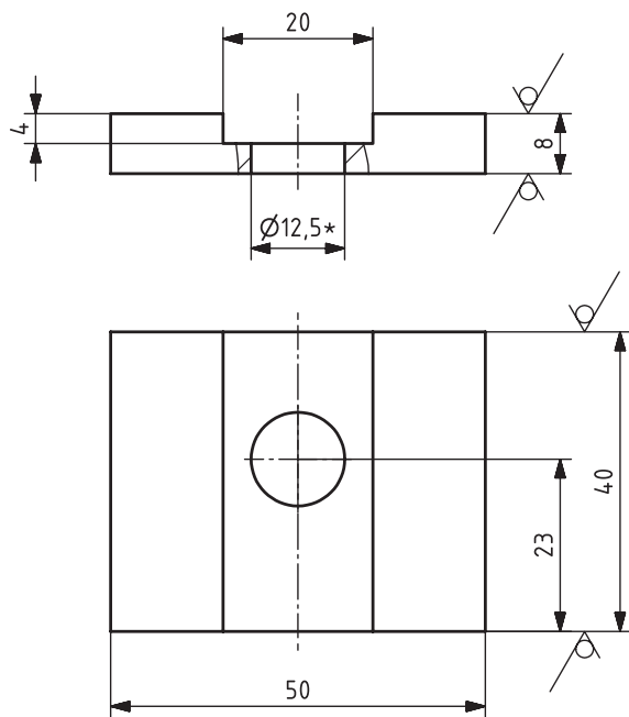
Skizze 21 \sqrt{Rz\ 16} (✓)
