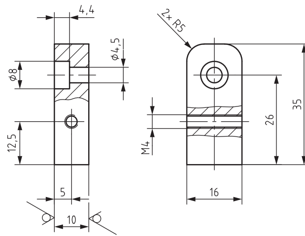
Skizze 13 \sqrt{Rz\ 16} (✓)
