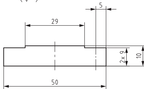
Skizze 14 \sqrt{Rz\ 16} (✓)
