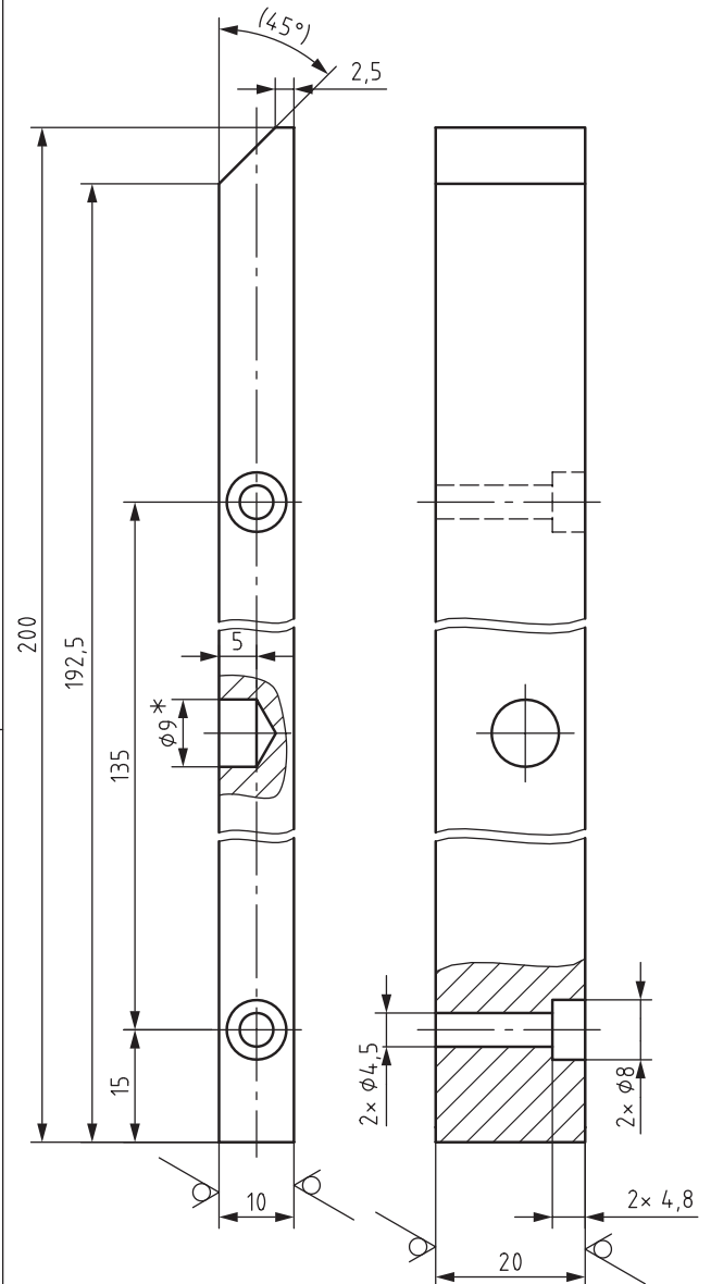
Skizze 8.2.1 \sqrt{Rz\ 16} (✓)
