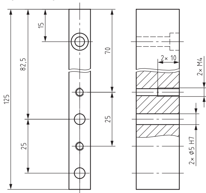
Skizze 8.1.2 \sqrt{Rz\ 16} (✓)
