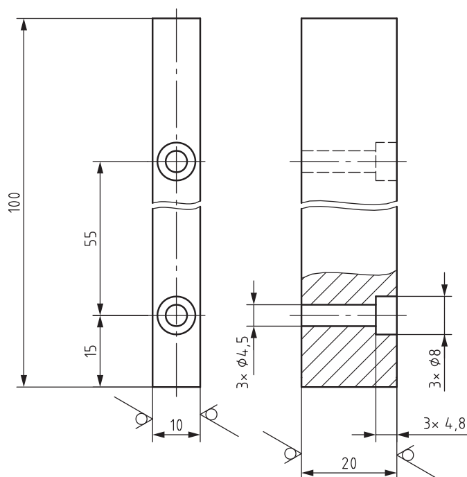
Skizze 8.1.2 \sqrt{Rz\ 16} (✓)
