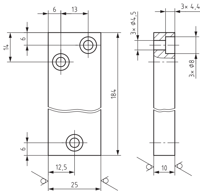
Skizze 2 \sqrt{Rz\ 16} (✓)
