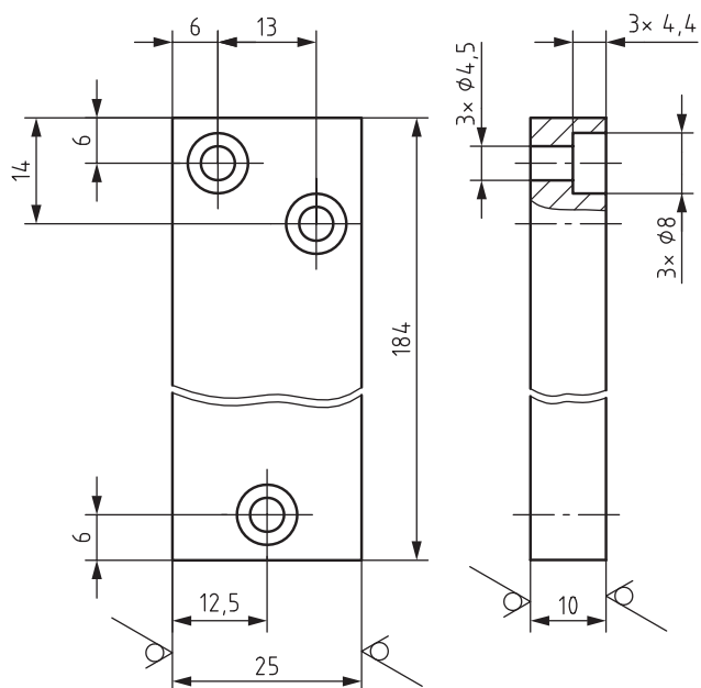
Skizze 1 \sqrt{Rz\ 16} (✓)
