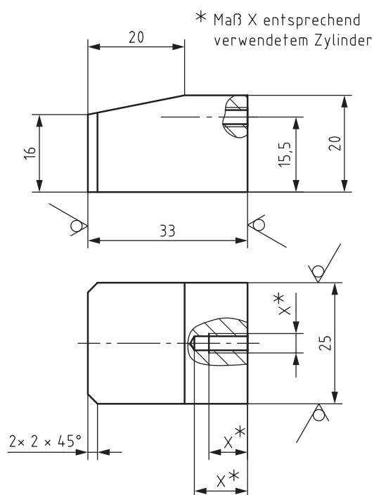
Skizze 5 \sqrt{Rz\ 16} (✓)
