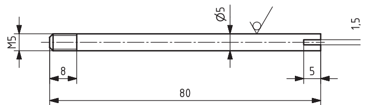
Skizze 23 \sqrt{Rz\ 16} (✓)
