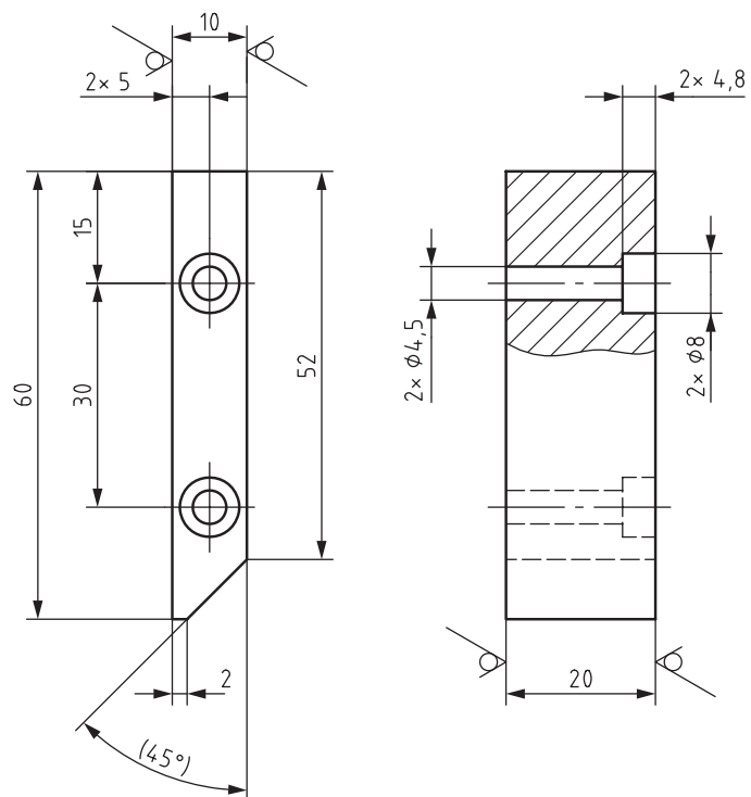
Skizze 8.4 \sqrt{Rz\ 16} (✓)
