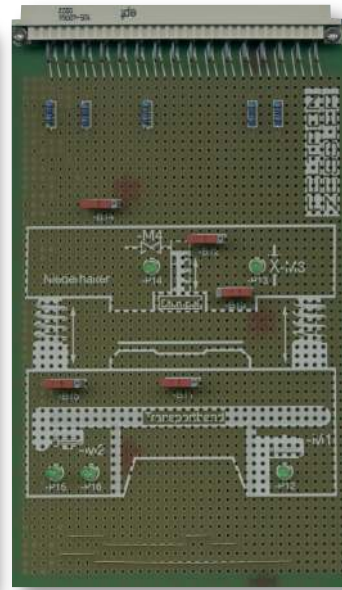
Herbst 2023 Platine Prozesssimulation 5035-1438
