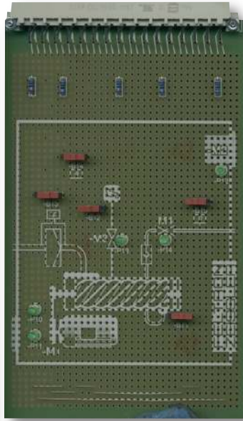
Frühjahr 2024 Platine Prozesssimulation 5035-1449
