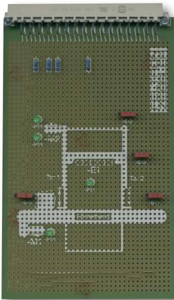
Herbst 2024 Platine Prozesssimulation 5035-1462
