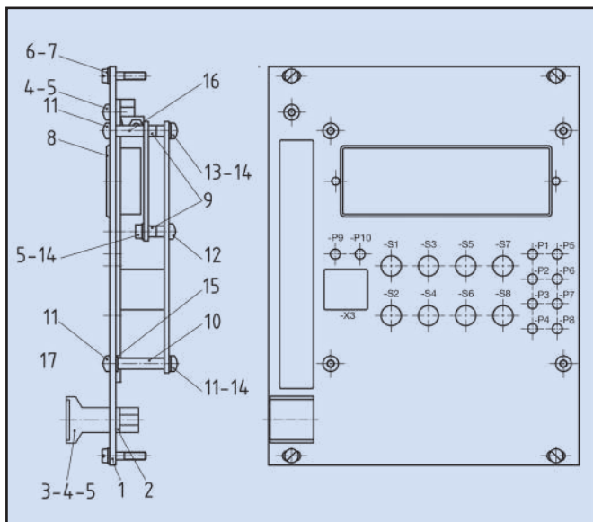
Bausatz Einschub 5035-1363
